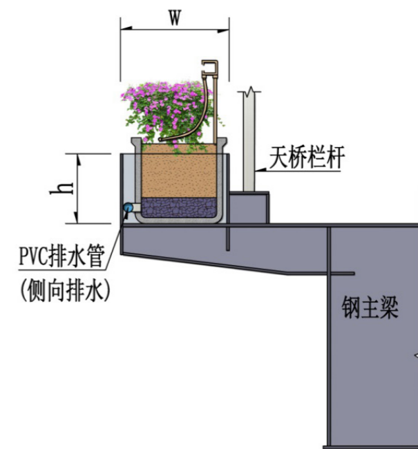
图 6.04 钢结构天桥搁置式花盆大样
