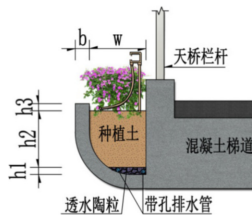
图 6.05 混凝土梯道一体式种植槽大样
