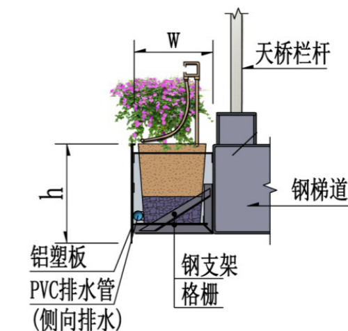
图 6.06 钢结构梯道悬挂式种植槽大样
